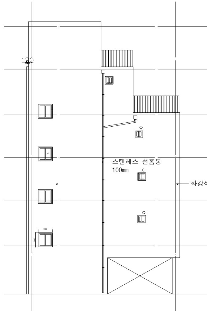
1 배면도 축척 : 1/100
