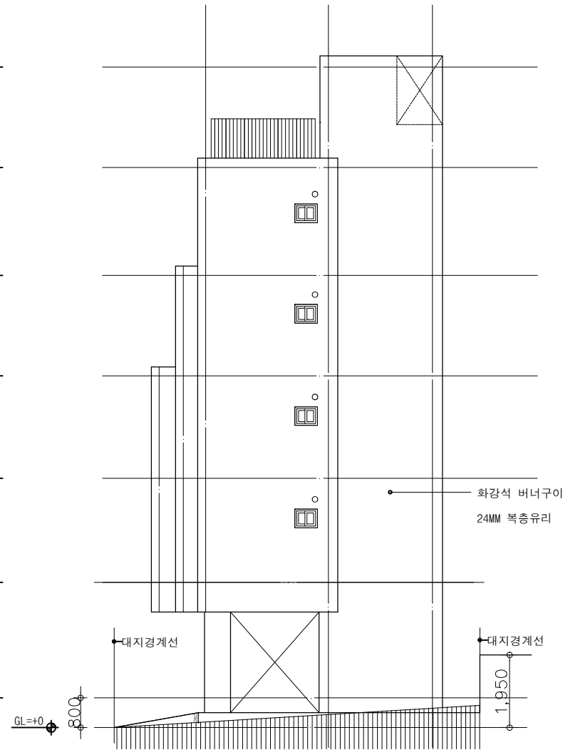
1 우측면도 축척 : 1/100
